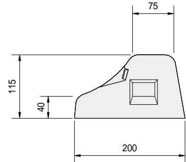
側面図
