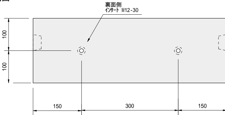
底面図
